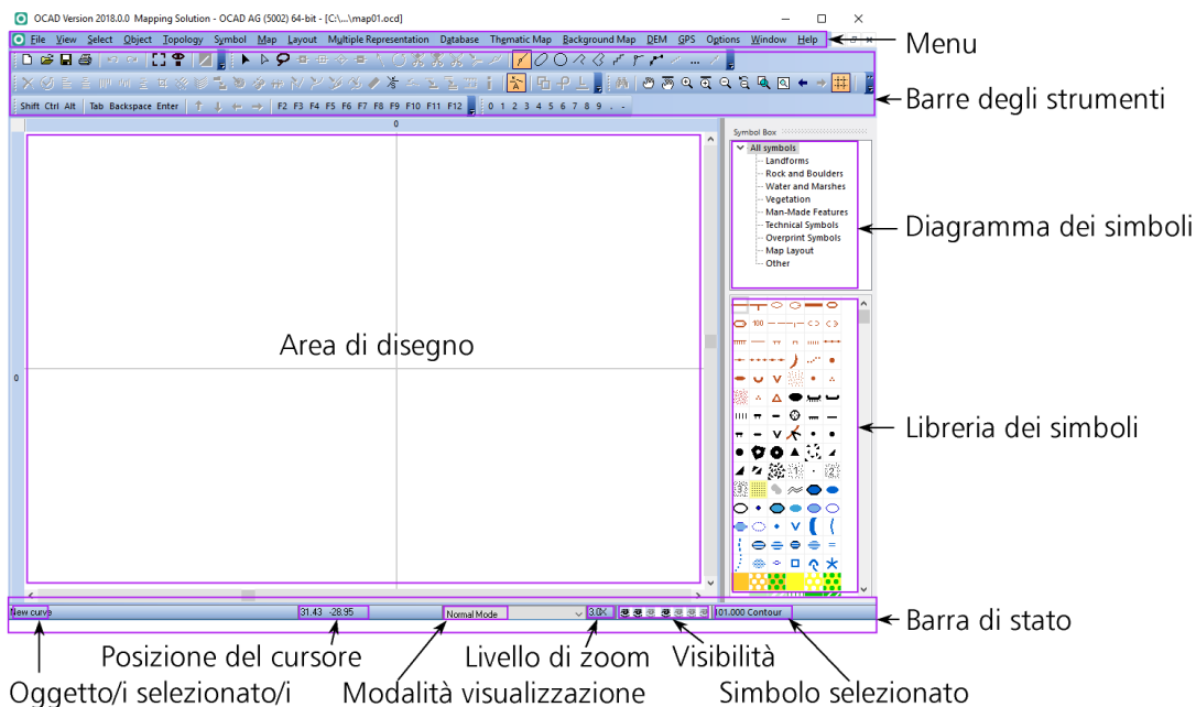
Fig. 1: Interfaccia grafica con menu, barre degli strumenti, area di disegno, barra di stato, diagramma dei simboli e libreria dei simboli.
