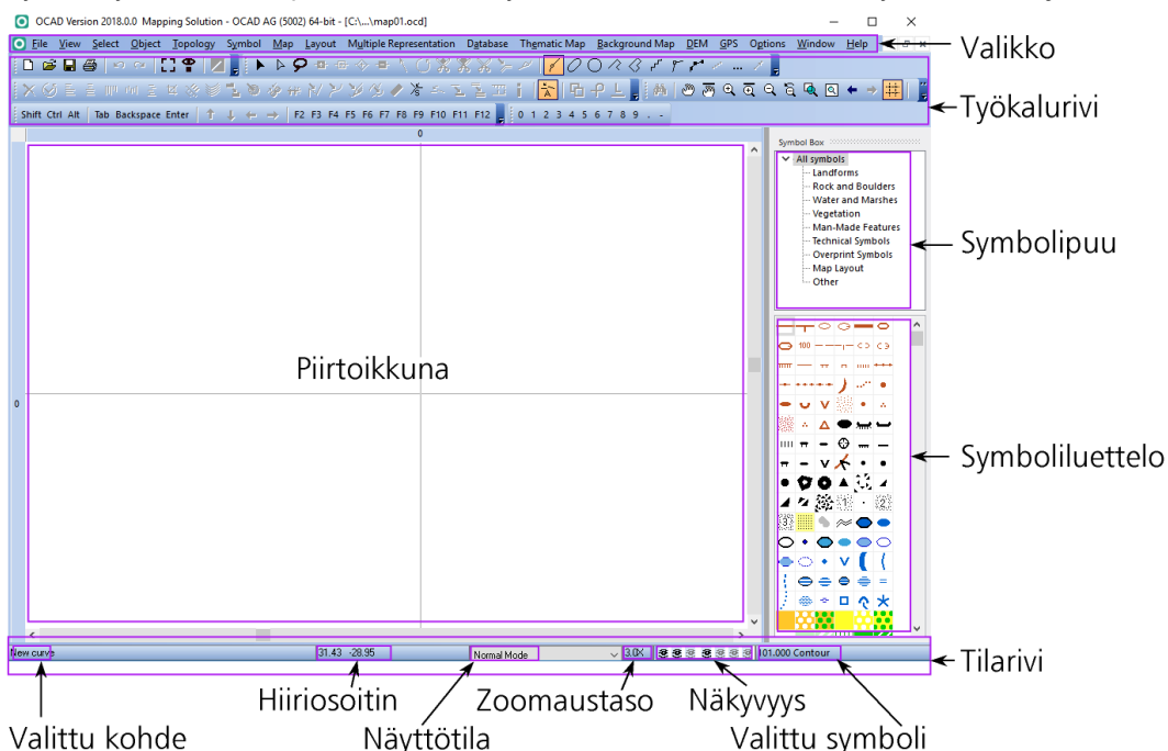
Kuva. 1: Käyttöliittymä, jossa on valikko, työkalurivi, piirtoikkuna, tilarivi, symbolipuu ja symboliluettelo
